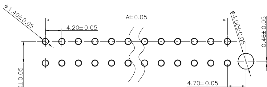
P.C.B LAYOUT TOLERANCE±0.05
