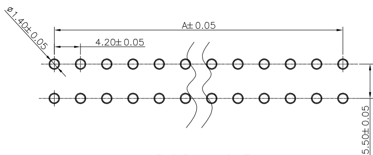
P.C.B LAYOUT TOLERANCE±0.05
