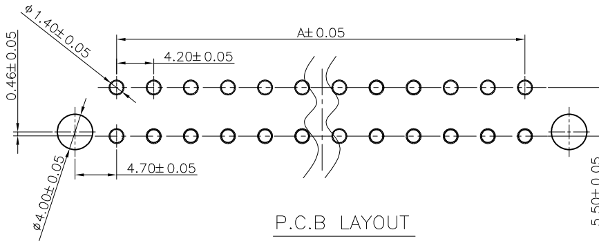
34202W07-2XNPx-Dx-xx: 左右耳规格PCB LAYOUT
