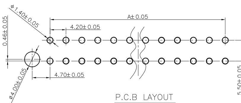
34202W07-2XNPx-Lx-xx: 左耳规格PCB LAYOUT
